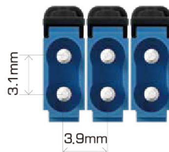
MDCコネクタ
